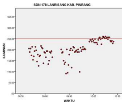
Gambar 7. Grafik Intensitas Cahaya Alami SDN 178 Lanrisang, Pinrang
