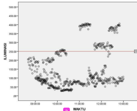
Gambar 8. Grafik Intensitas Cahaya Alami Ruang Kelas di Areal Pesisir Pantai Sulawesi Selatan
