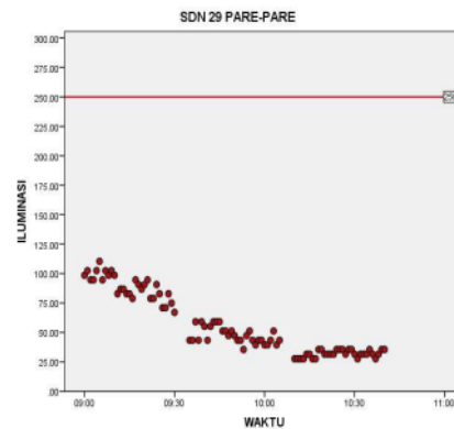
Gambar 5. Grafik Intensitas Cahaya Alami SD Negeri 29 Kota Pare-Pare
